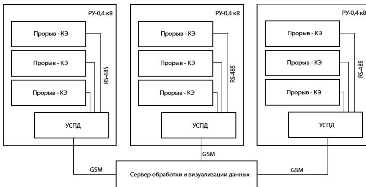
Рис. 2. Структура системы мониторинга качества электроэнергии
