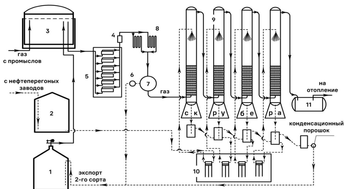
1 – резервуар с бензином; 2 – резервуар с лигроином; 3 – газгольдер; 4 – маслоотделитель; 5 – компрессорная станция; 6 – конденсированный порошок; 7 – генератор; 8 – холодильник; 9 – скрубберы; 10 – насосное отделение; 11 – аккумулятор газа.
